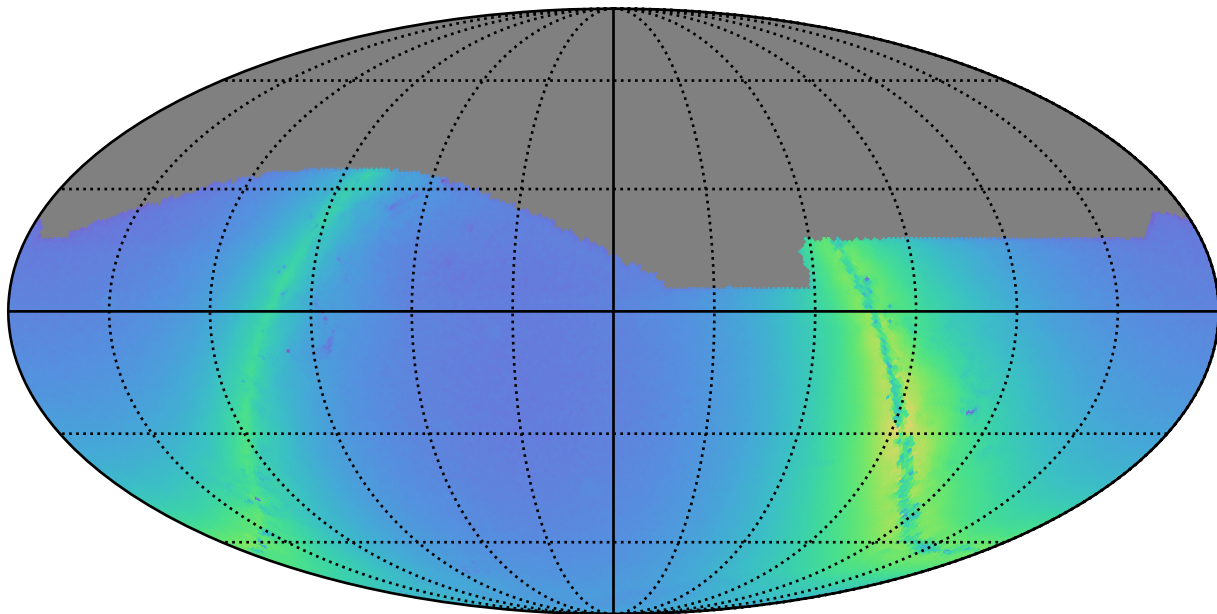
extra_ss_neo5_v3.4_10yrs r: Nstars_no_crowding
