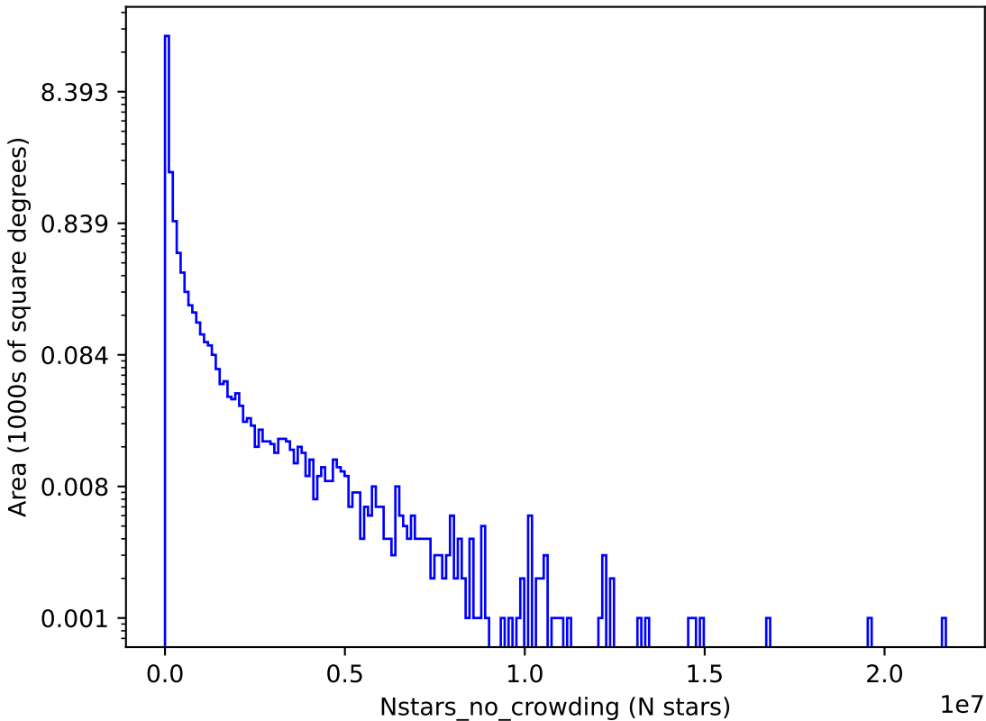
extra_ss_neo5_v3.4_10yrs r: Nstars_no_crowding
