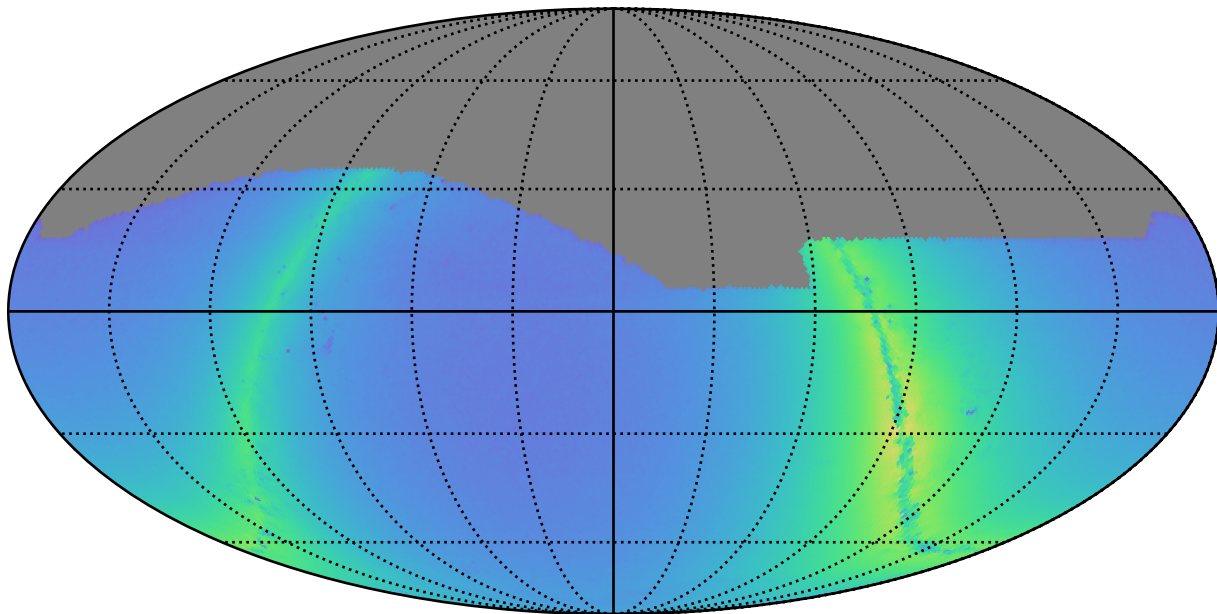
extra_ss_neo5_v3.4_10yrs i: Nstars_no_crowding
