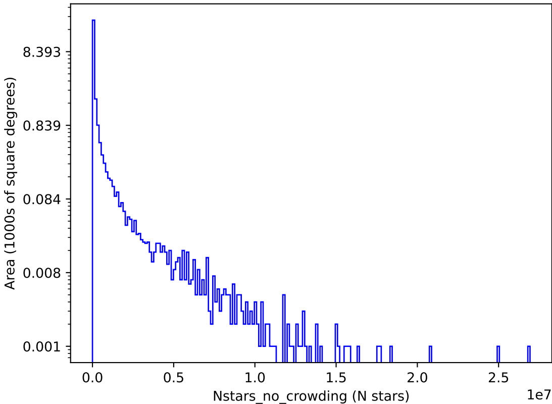
extra_ss_neo5_v3.4_10yrs i: Nstars_no_crowding
