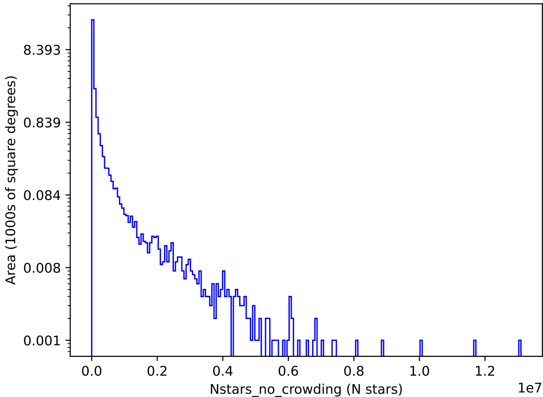
extra_ss_neo5_v3.4_10yrs g: Nstars_no_crowding
