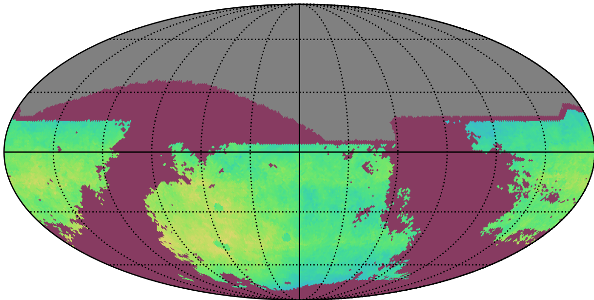
extra_ss_neo5_v3.4_10yrs i: NgalScale
