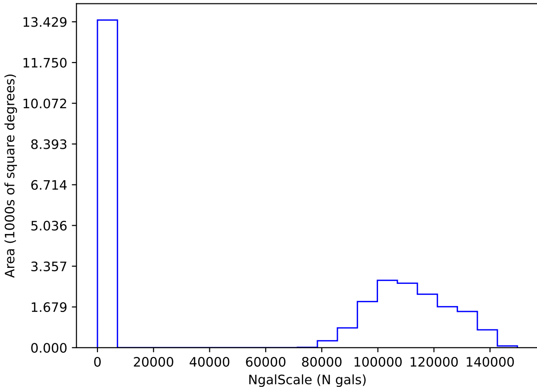
extra_ss_neo5_v3.4_10yrs i: NgalScale
