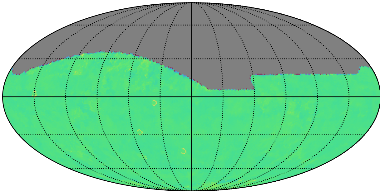
extra_ss_neo5_v3.4_10yrs z: Kuiper rotTelPos
