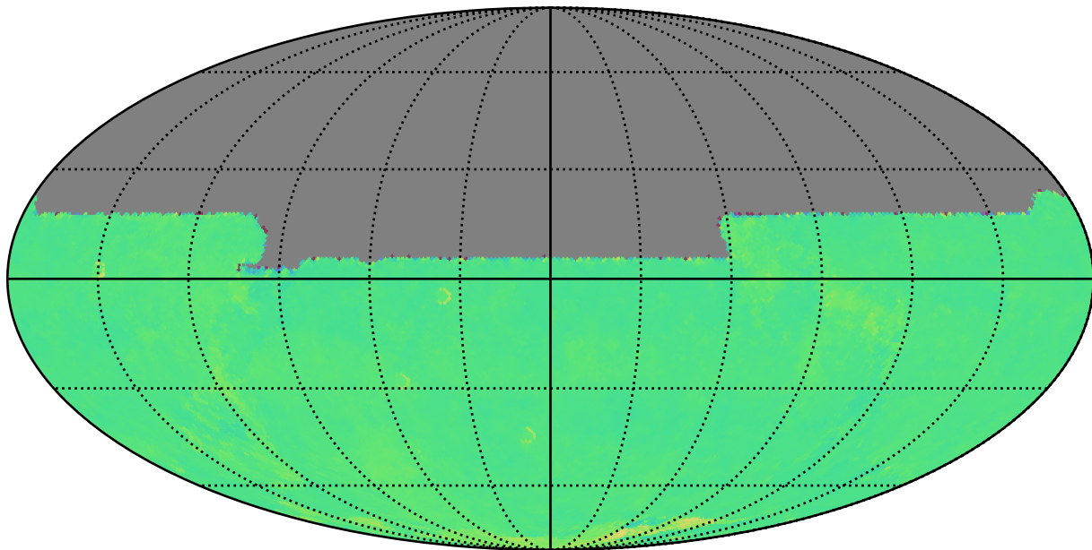
extra_ss_neo5_v3.4_10yrs y: Kuiper rotTelPos
