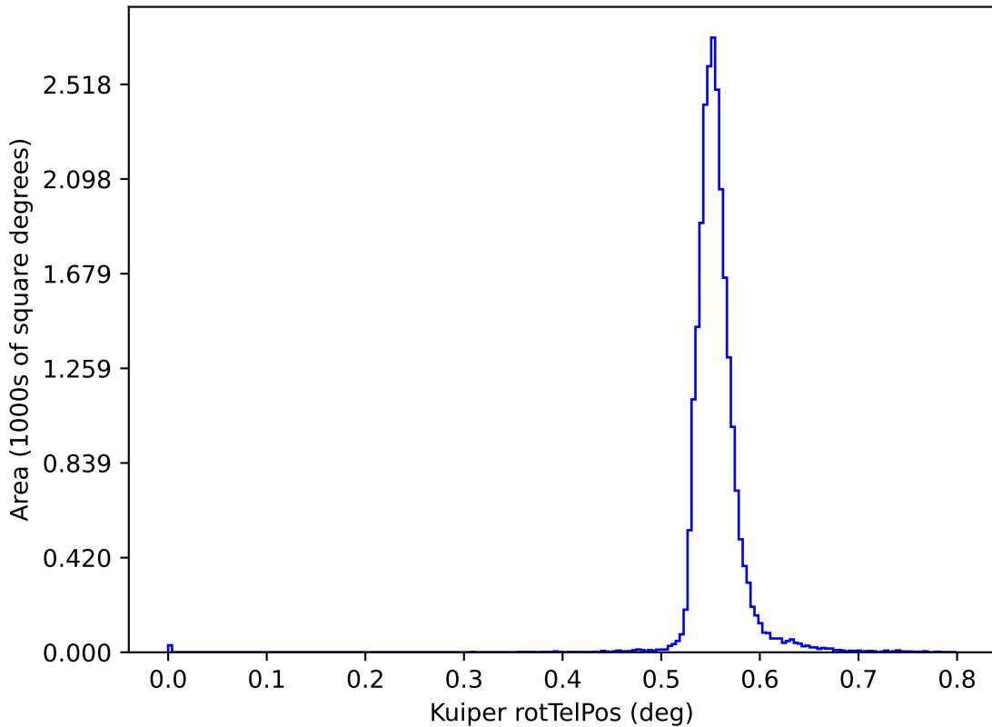
extra_ss_neo5_v3.4_10yrs y: Kuiper rotTelPos
