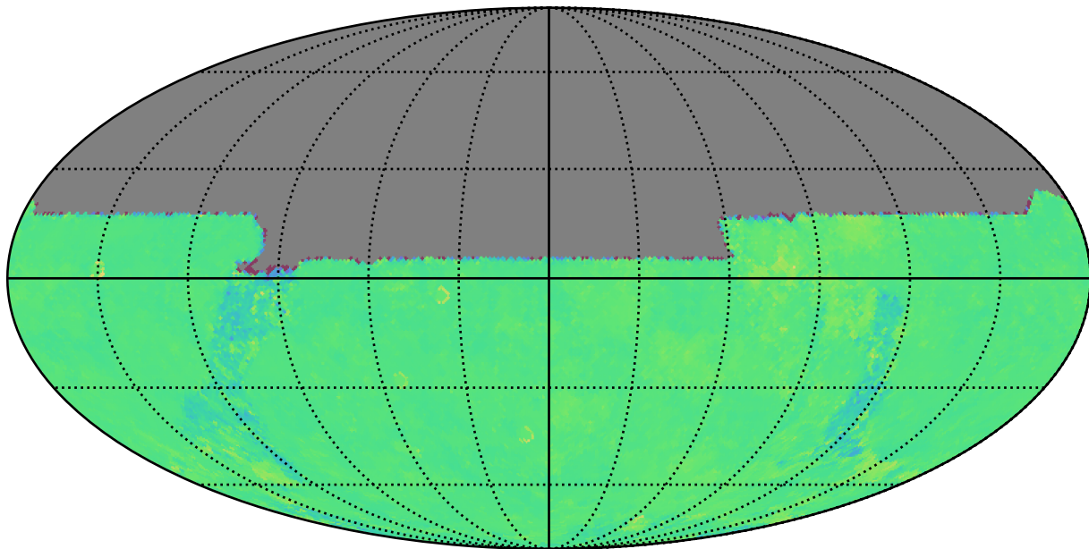
extra_ss_neo5_v3.4_10yrs u: Kuiper rotTelPos
