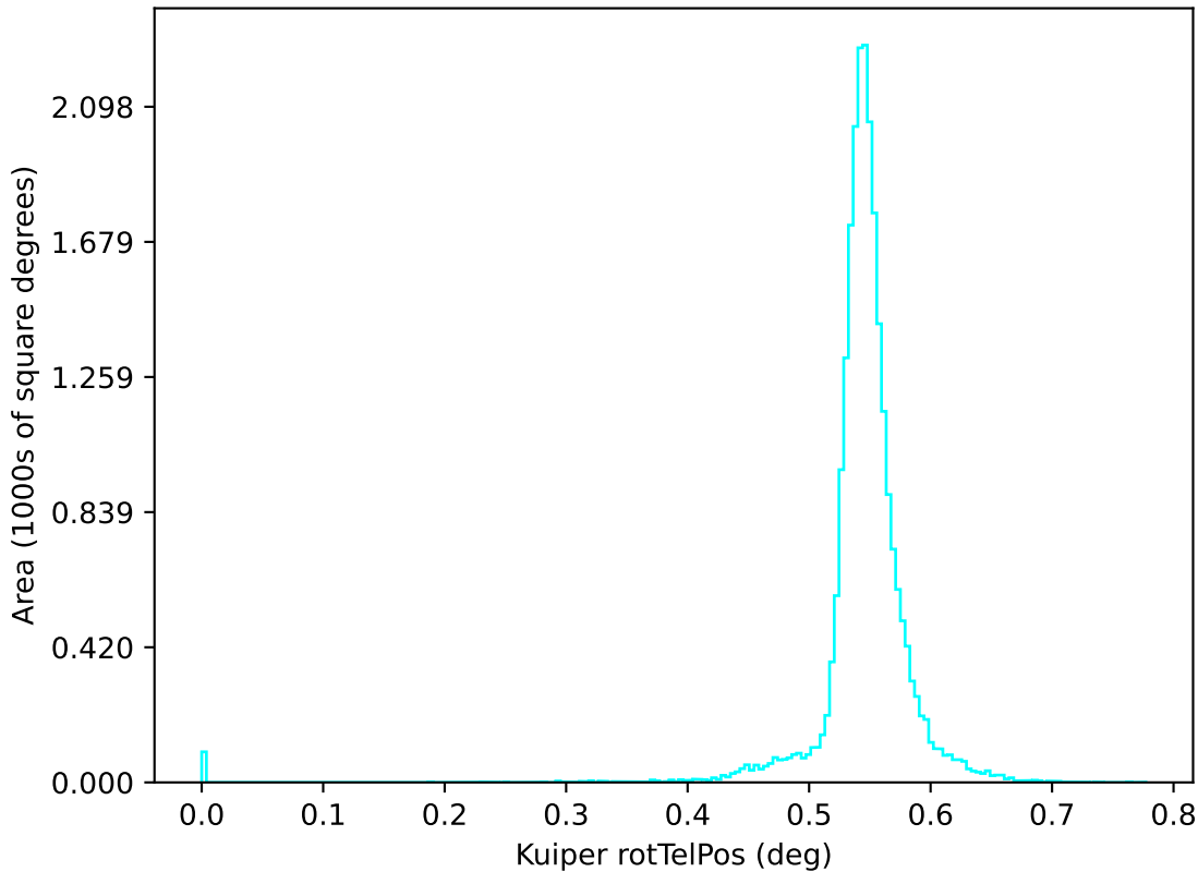
extra_ss_neo5_v3.4_10yrs u: Kuiper rotTelPos
