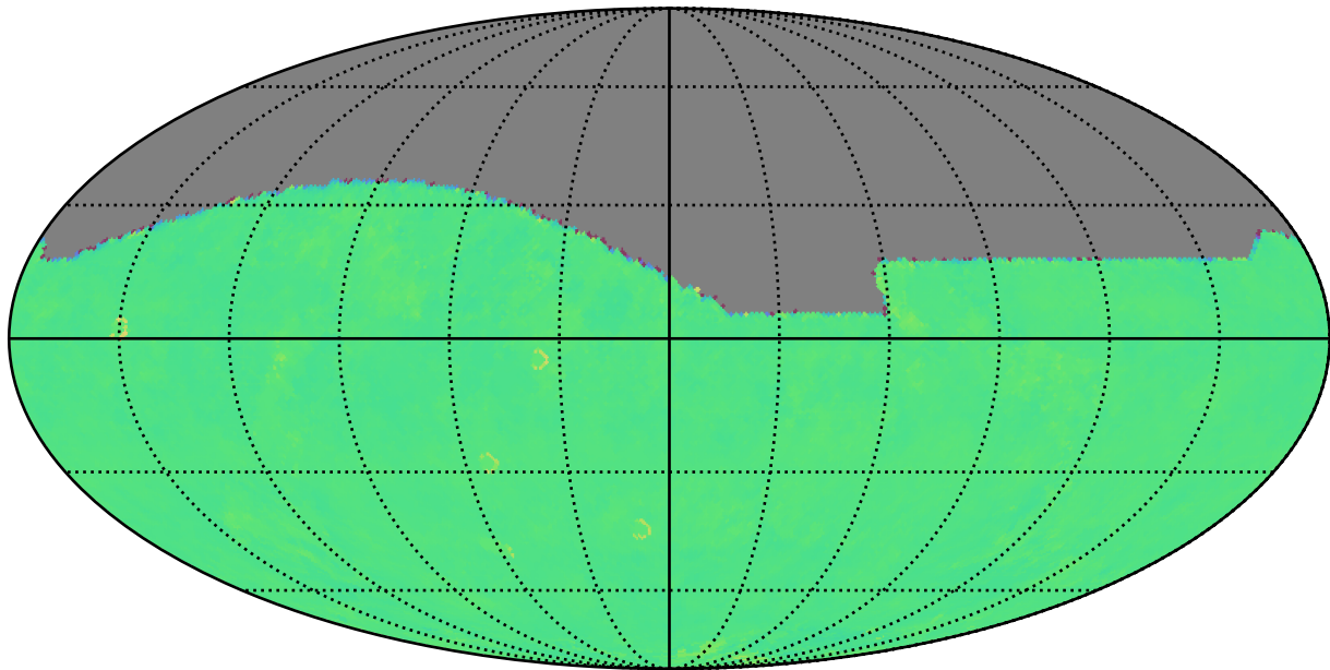
extra_ss_neo5_v3.4_10yrs r: Kuiper rotTelPos
