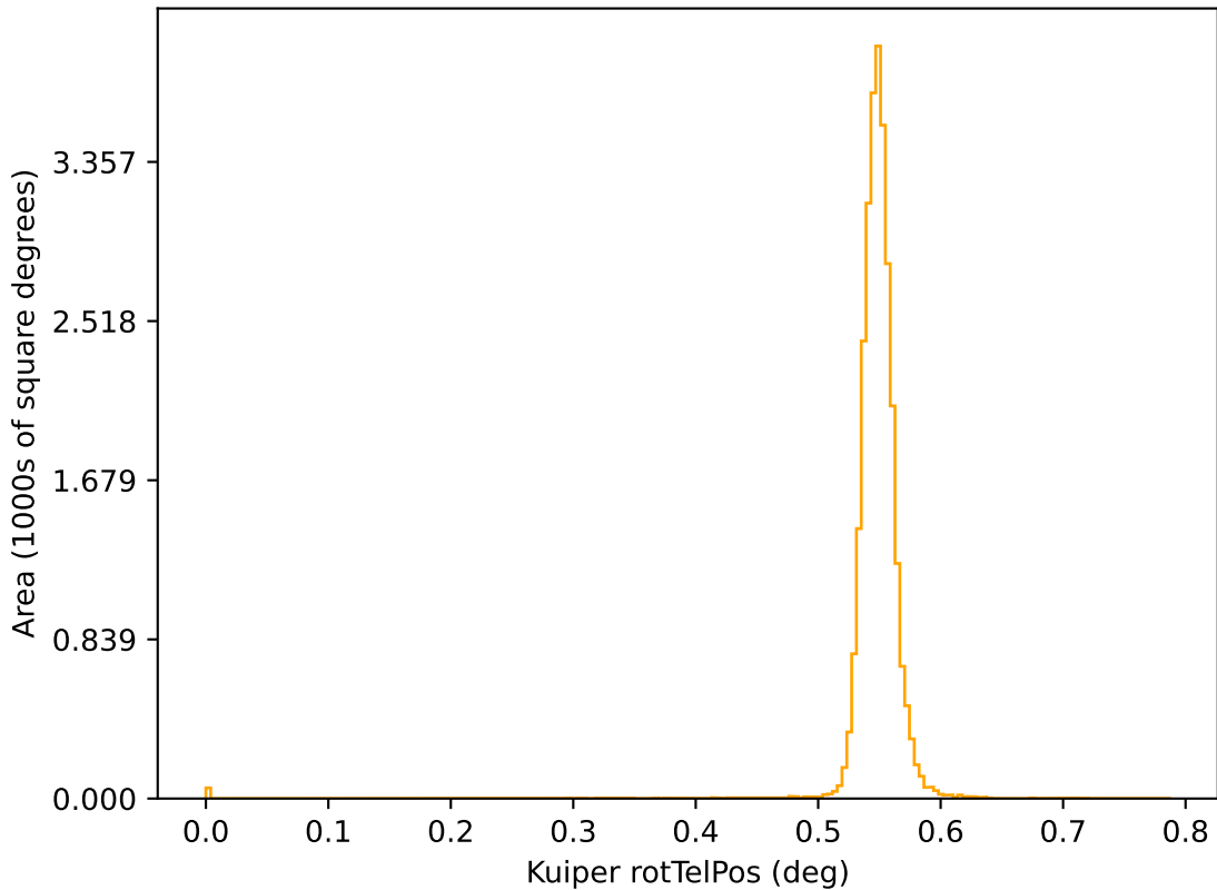
extra_ss_neo5_v3.4_10yrs r: Kuiper rotTelPos
