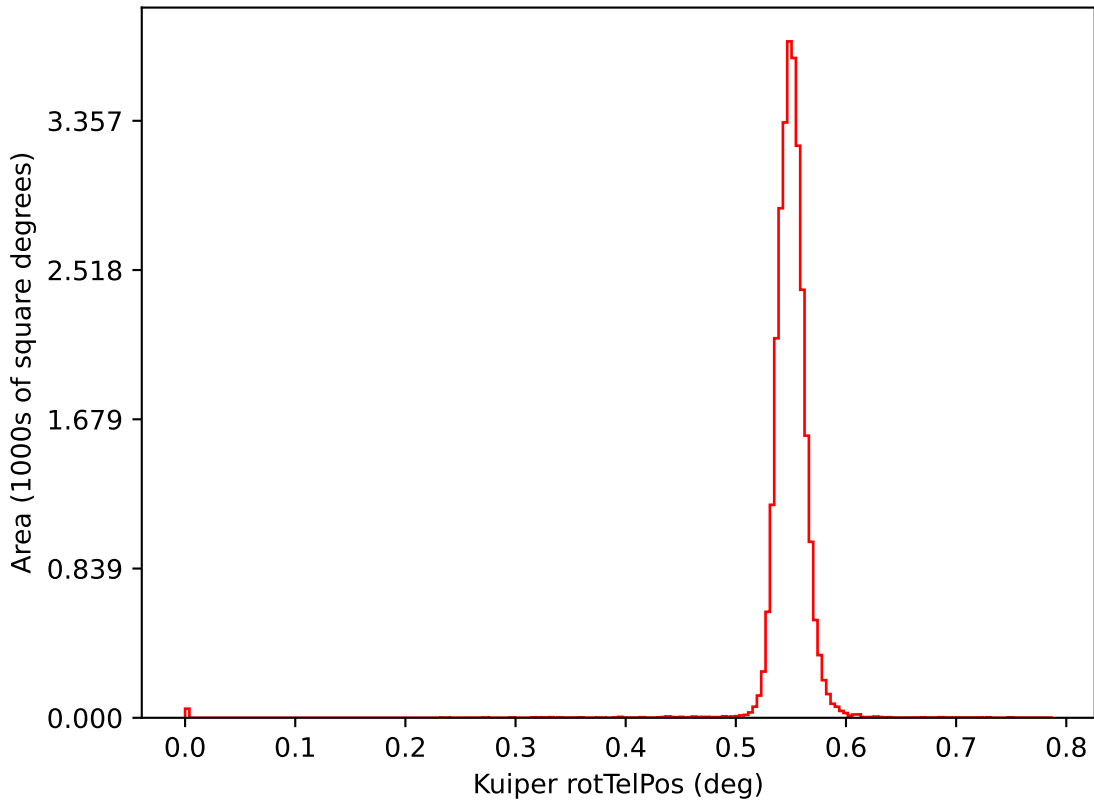
extra_ss_neo5_v3.4_10yrs i: Kuiper rotTelPos
