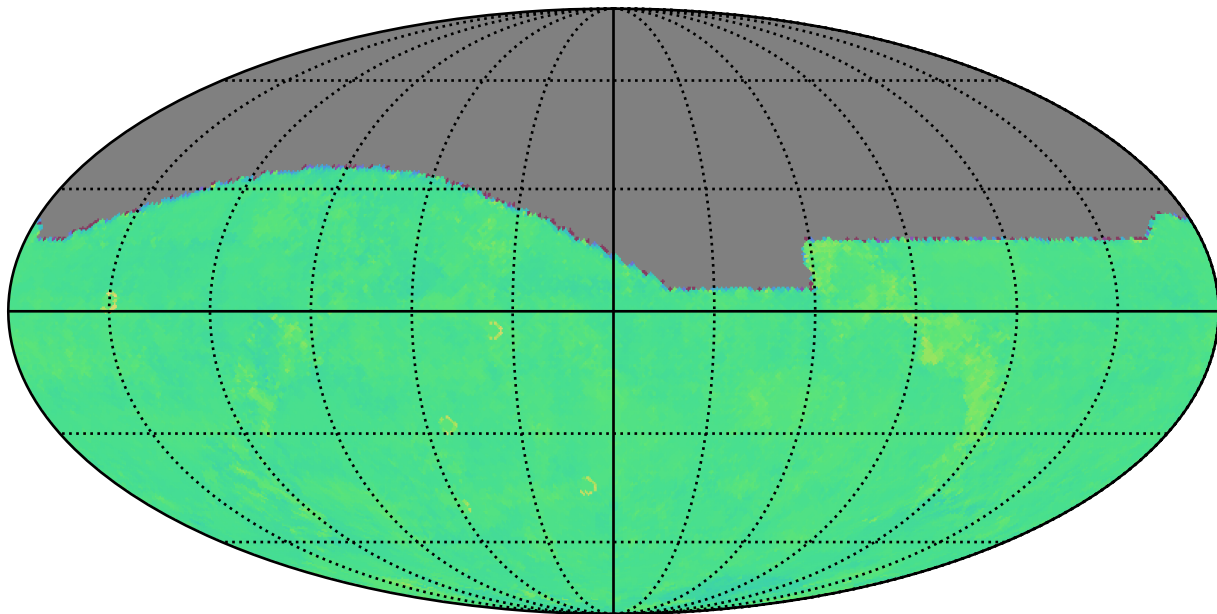
extra_ss_neo5_v3.4_10yrs g: Kuiper rotTelPos
