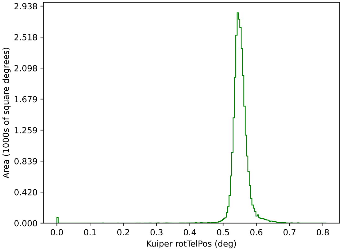
extra_ss_neo5_v3.4_10yrs g: Kuiper rotTelPos
