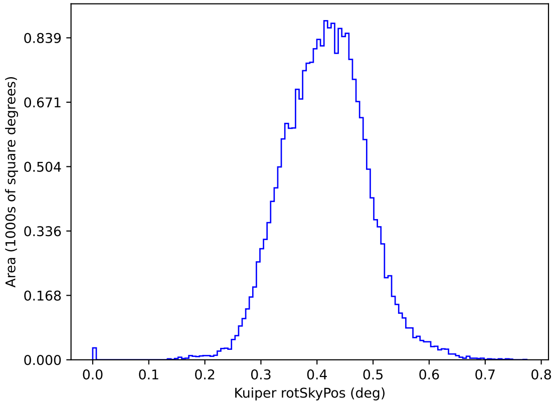
extra_ss_neo5_v3.4_10yrs y: Kuiper rotSkyPos
