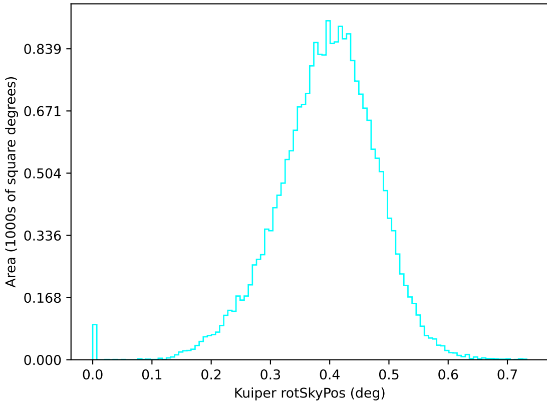
extra_ss_neo5_v3.4_10yrs u: Kuiper rotSkyPos
