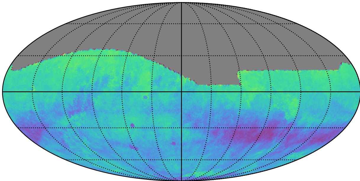
extra_ss_neo5_v3.4_10yrs r: Kuiper rotSkyPos
