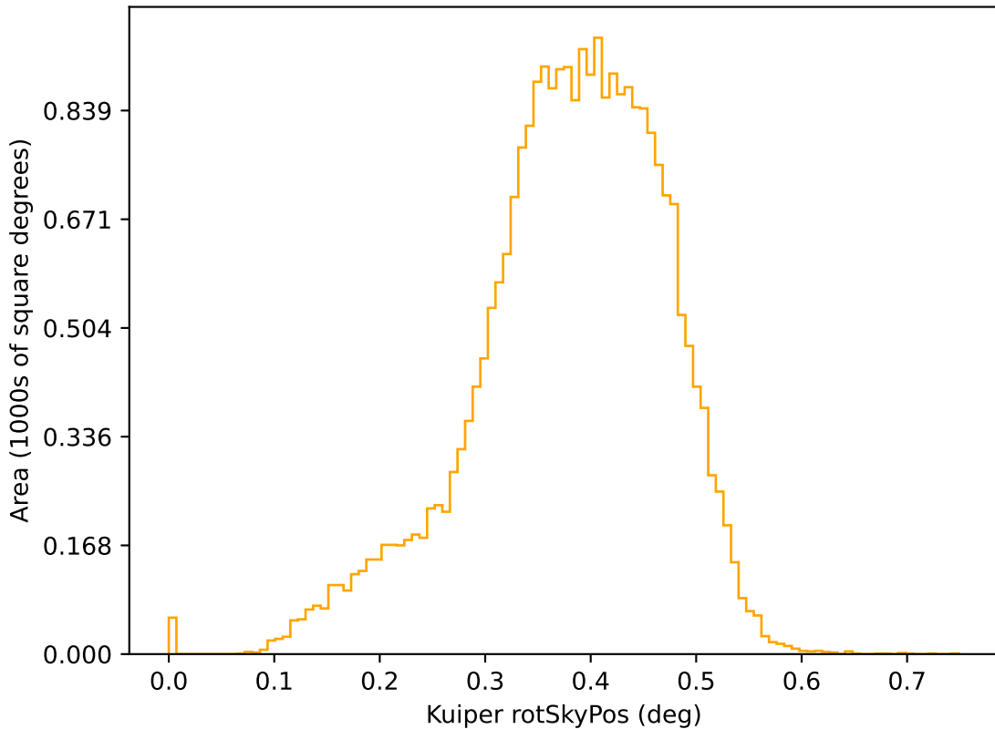
extra_ss_neo5_v3.4_10yrs r: Kuiper rotSkyPos
