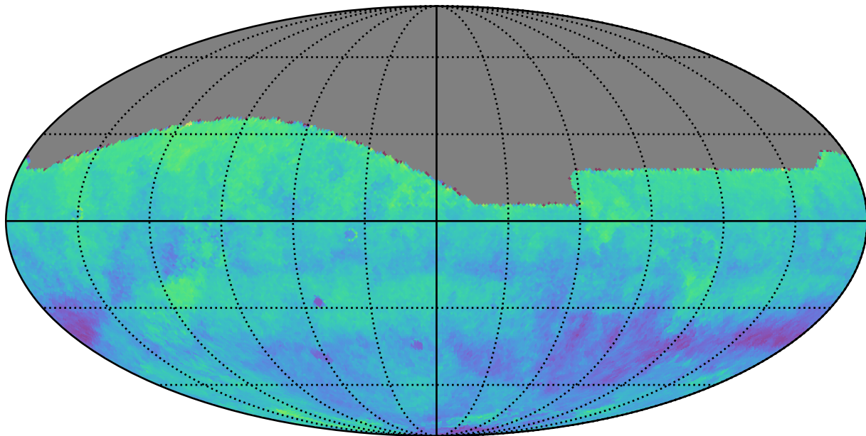
extra_ss_neo5_v3.4_10yrs i: Kuiper rotSkyPos
