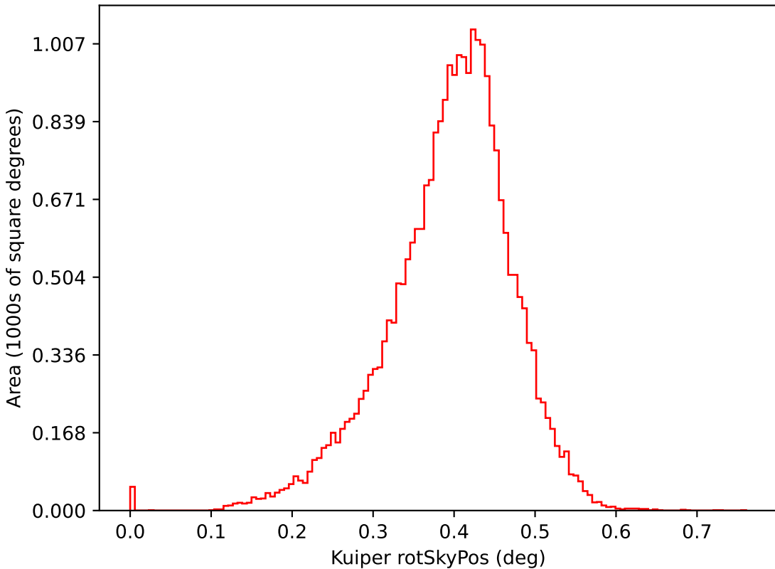
extra_ss_neo5_v3.4_10yrs i: Kuiper rotSkyPos
