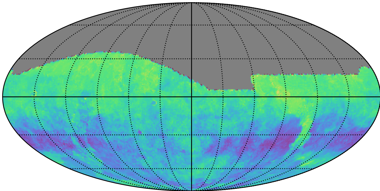
extra_ss_neo5_v3.4_10yrs g: Kuiper rotSkyPos
