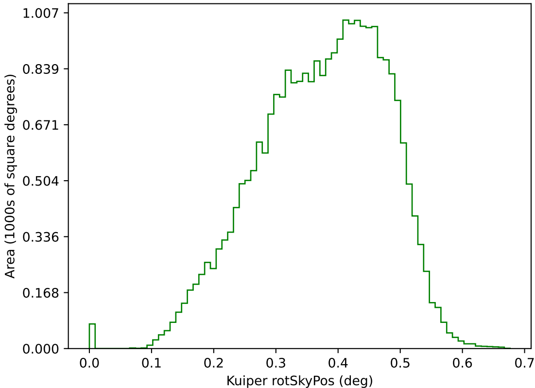
extra_ss_neo5_v3.4_10yrs g: Kuiper rotSkyPos
