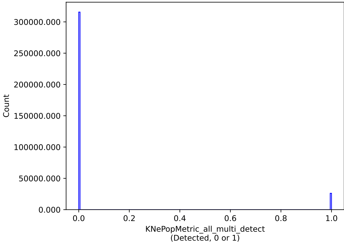
extra_ss_neo5_v3.4_10yrs all models: KNePopMetric_all_multi_detect
