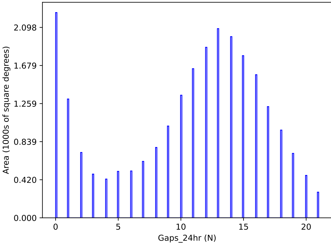
extra_ss_neo5_v3.4_10yrs y band: Gaps_24hr
