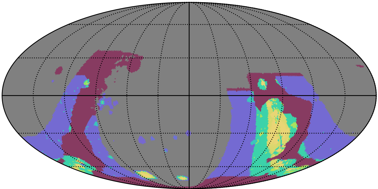
extra_ss_neo5_v3.4_10yrs : GalplaneFootprintMetric_combined_map_Tau_11_0
