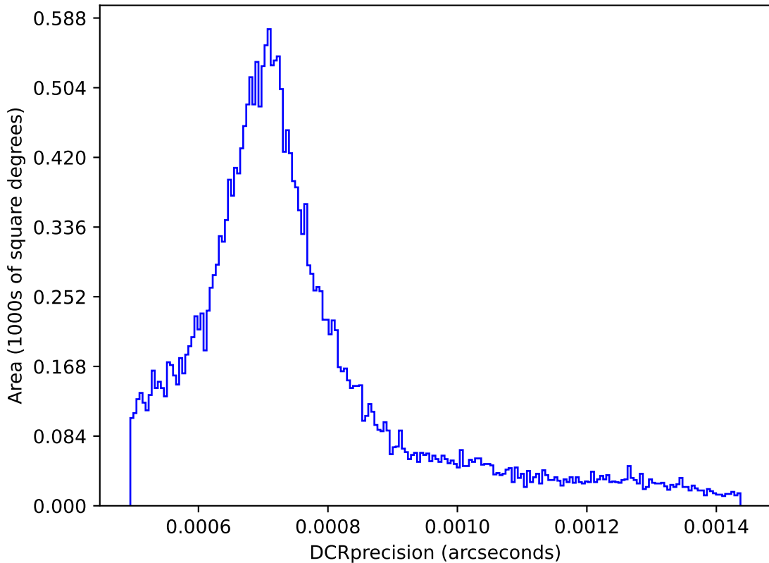
extra_ss_neo5_v3.4_10yrs : DCRprecision
