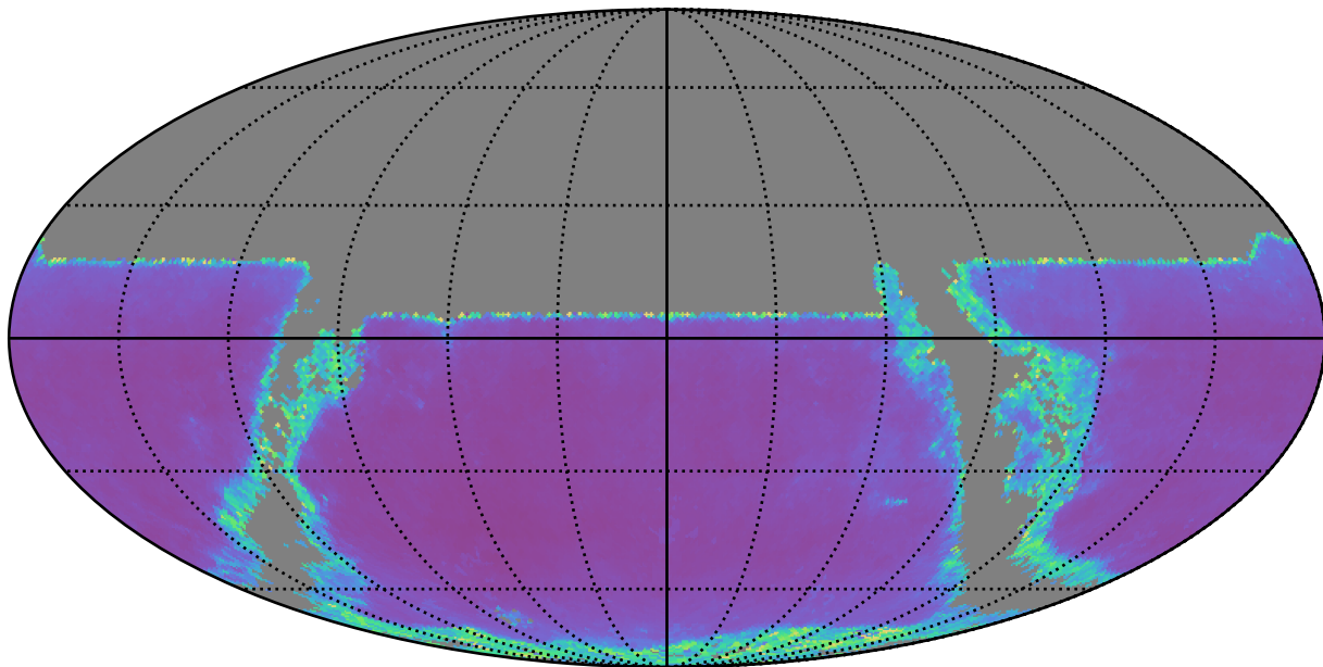
extra_ss_neo5_v3.4_10yrs y band: AGN SF_uncert
