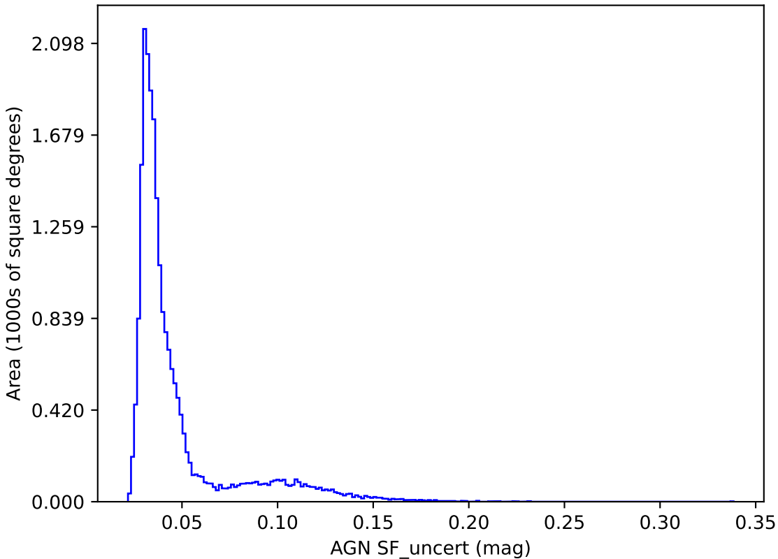
extra_ss_neo5_v3.4_10yrs y band: AGN SF_uncert
