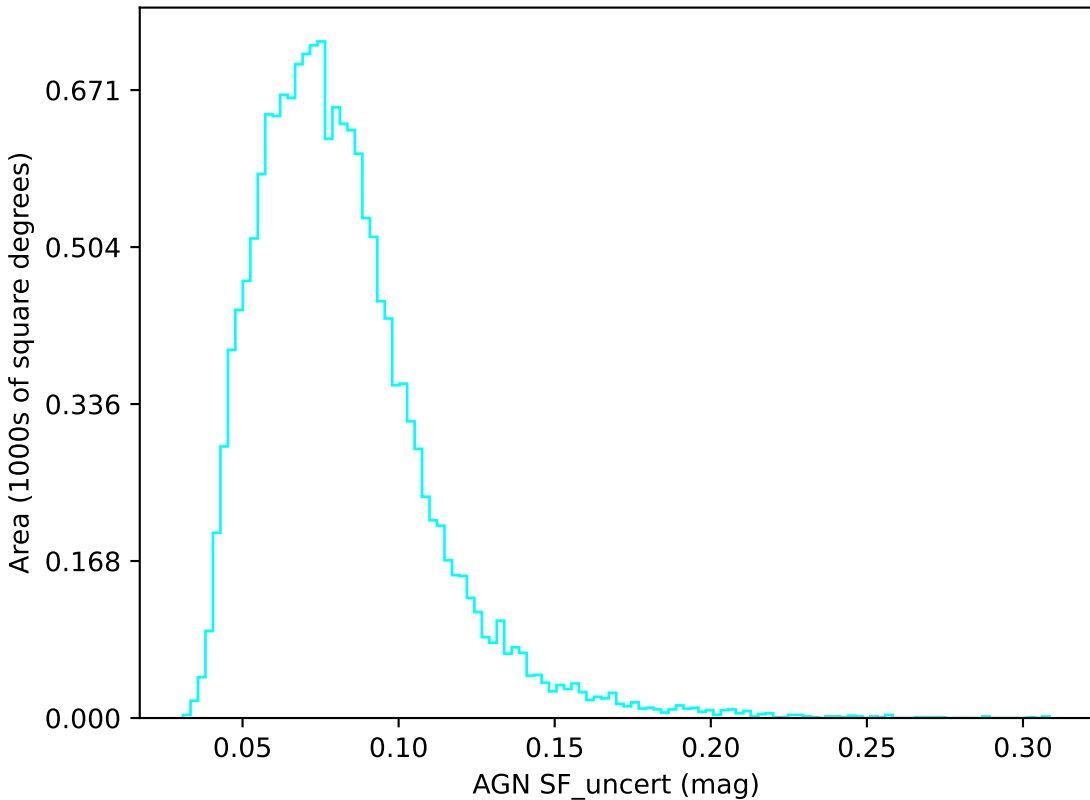
extra_ss_neo5_v3.4_10yrs u band: AGN SF_uncert
