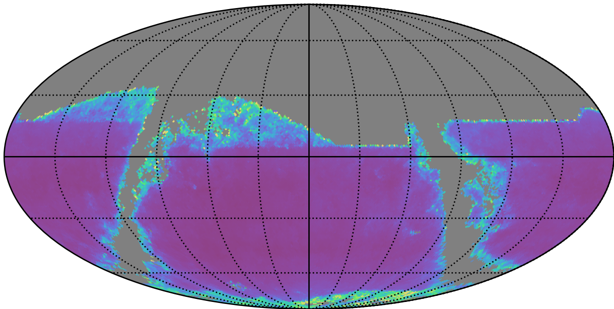
extra_ss_neo5_v3.4_10yrs i band: AGN SF_uncert
