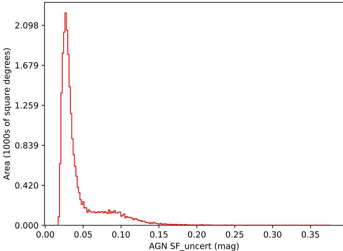
extra_ss_neo5_v3.4_10yrs i band: AGN SF_uncert
