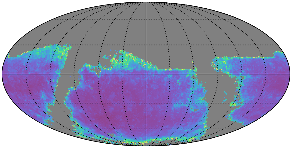
extra_ss_neo5_v3.4_10yrs g band: AGN SF_uncert
