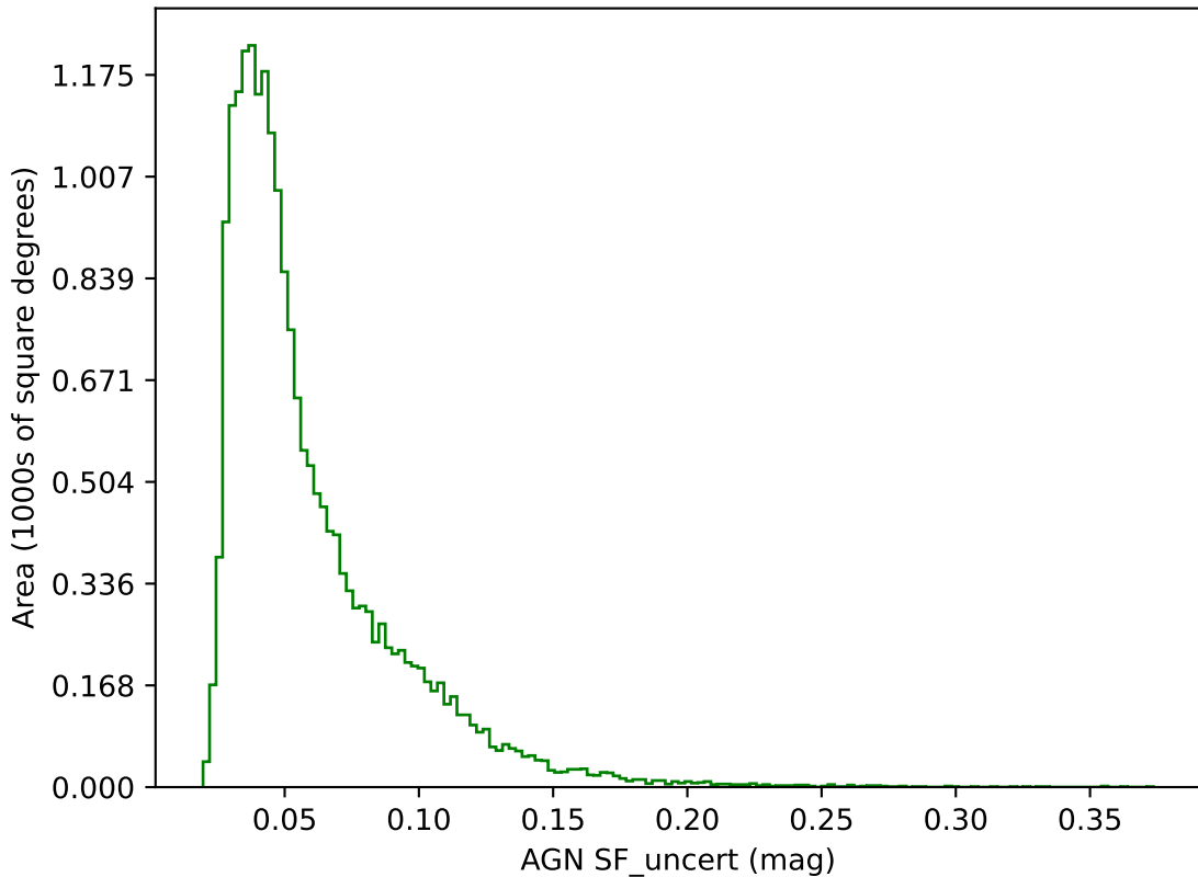
extra_ss_neo5_v3.4_10yrs g band: AGN SF_uncert
