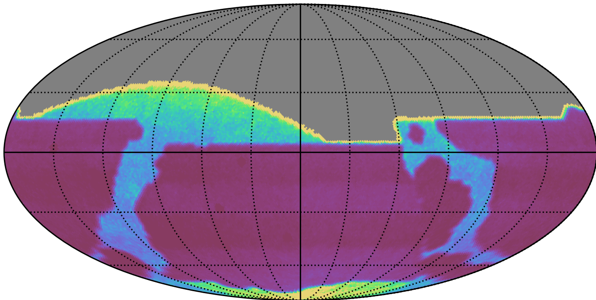
extra_ss_neo5_v3.4_10yrs : properMotion
