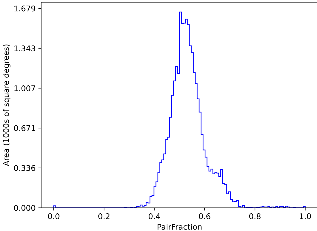
extra_ss_neo5_v3.4_10yrs (g or r or i): PairFraction
