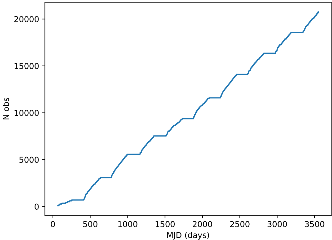
extra_ss_neo5_v3.4_10yrs note like DD:ELAISS1%: Cumulative
