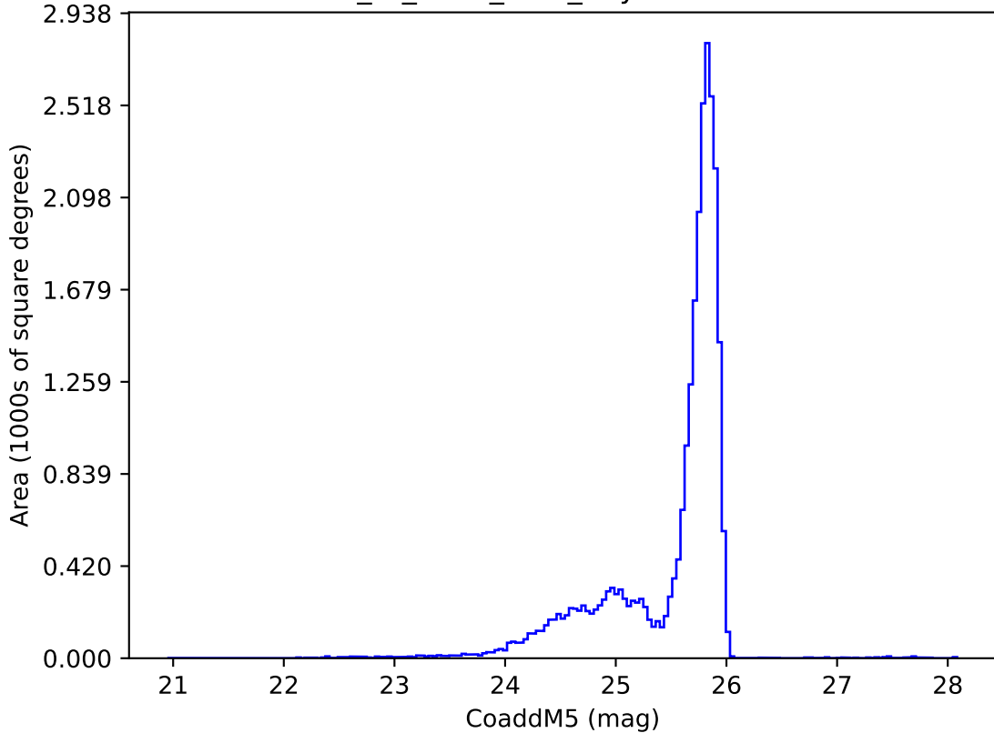
extra_ss_neo5_v3.4_10yrs z: CoaddM5
