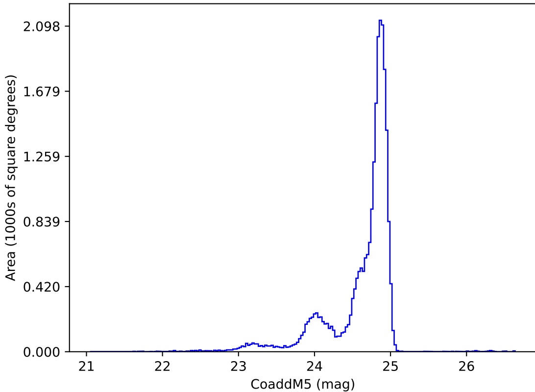
extra_ss_neo5_v3.4_10yrs y: CoaddM5
