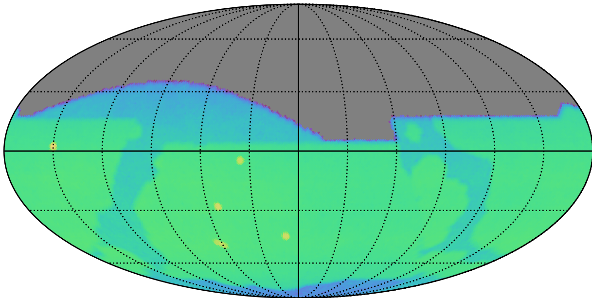
extra_ss_neo5_v3.4_10yrs r: CoaddM5
