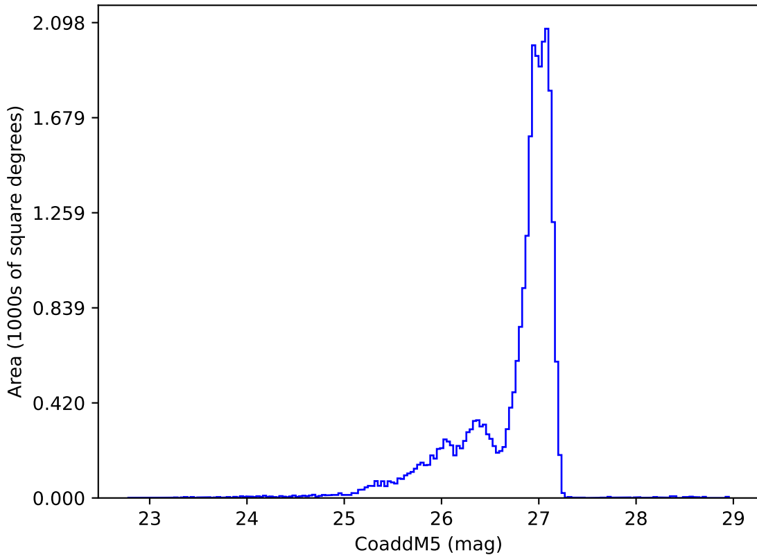
extra_ss_neo5_v3.4_10yrs r: CoaddM5
