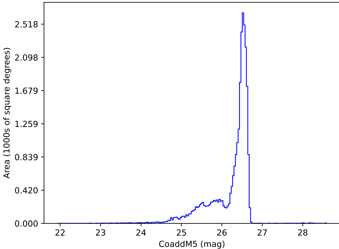
extra_ss_neo5_v3.4_10yrs i: CoaddM5
