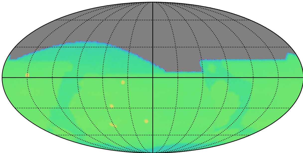
extra_ss_neo5_v3.4_10yrs : CoaddM5
