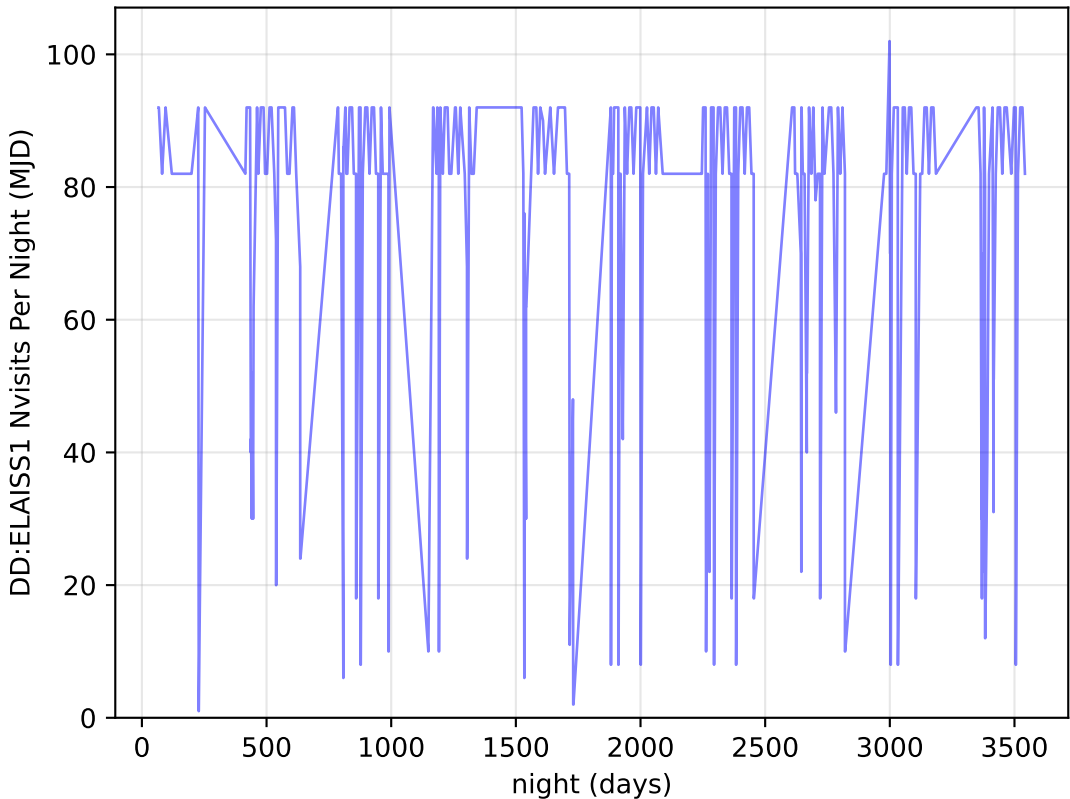
extra_ss_neo5_v3.4_10yrs all bands: DD:ELAISS1 Nvisits Per Night
