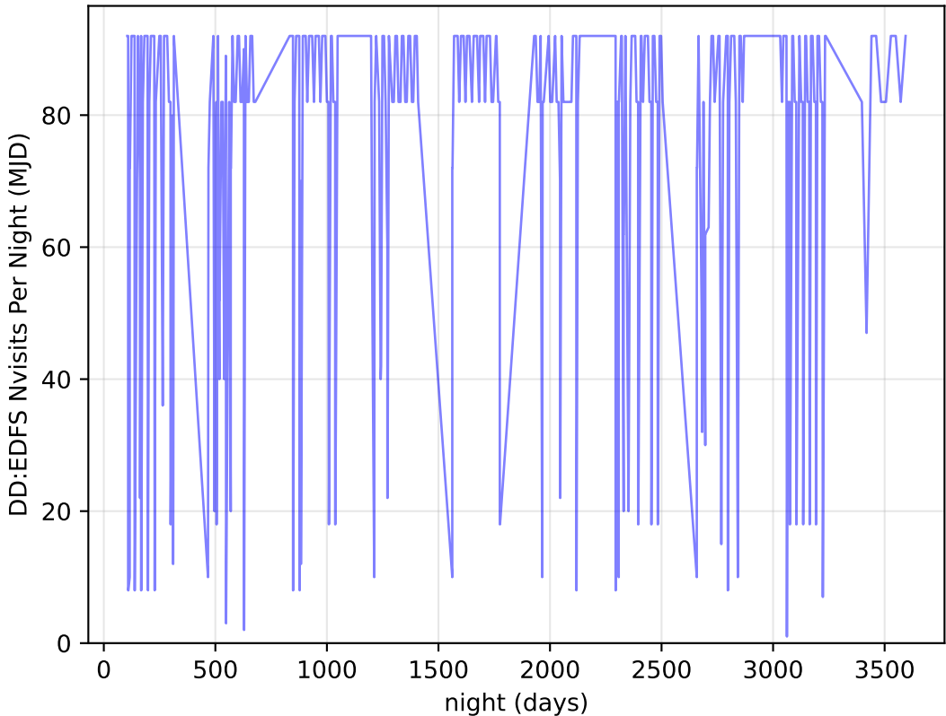
extra_ss_neo5_v3.4_10yrs all bands: DD:EDFS Nvisits Per Night
