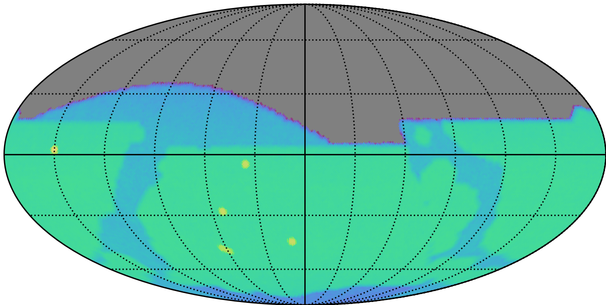
extra_ss_neo4_v3.4_10yrs i: SurfaceBrightLimit
