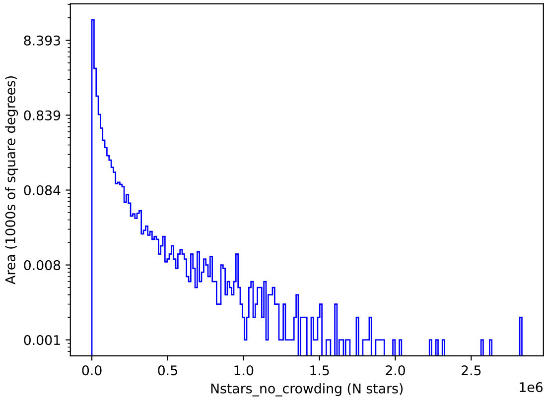
extra_ss_neo4_v3.4_10yrs u: Nstars_no_crowding
