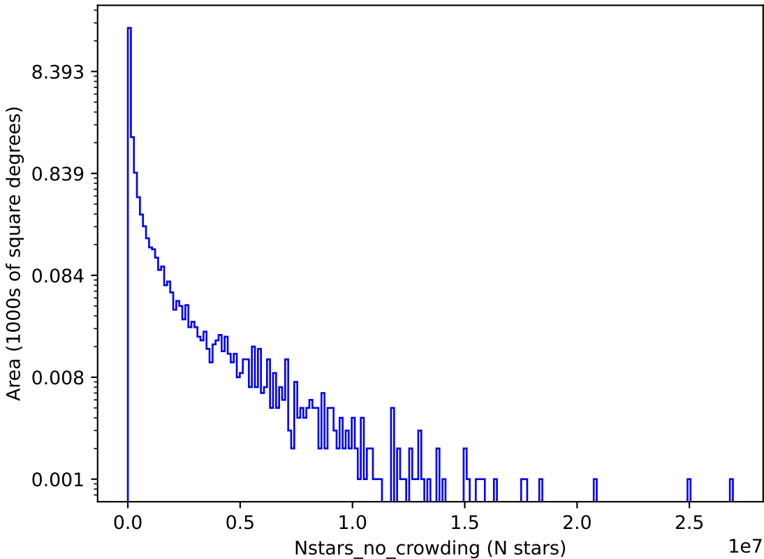
extra_ss_neo4_v3.4_10yrs i: Nstars_no_crowding
